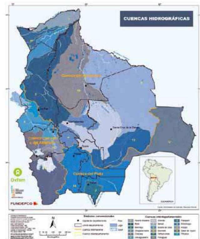
Mapa 8. Cuencas hidrográficas
