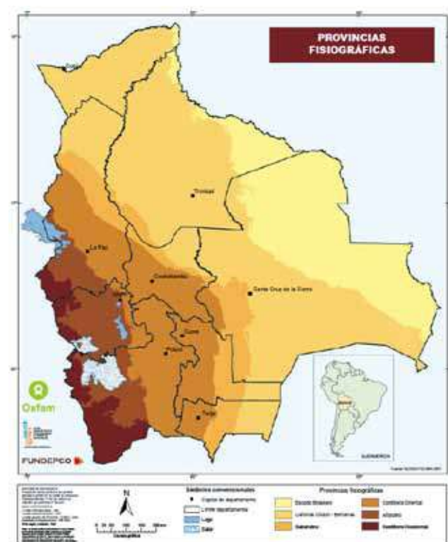
Mapa 1. Provincias Fisiográficas
