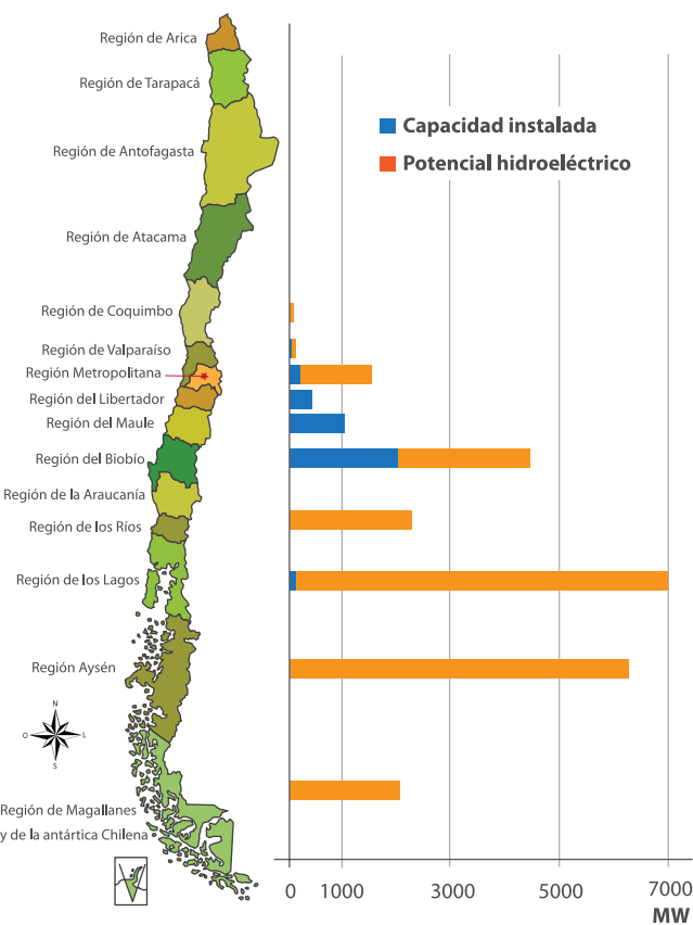
Figura 23. Potencial hidroeléctrico y capacidad instalada
