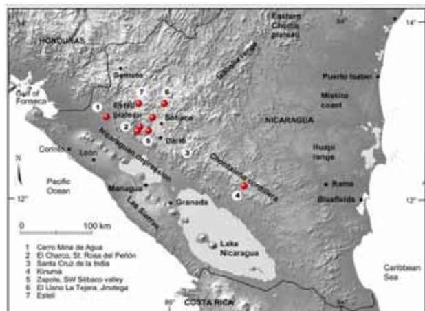
Figura 4.4. Ubicación de siete fuentes de agua potable con concentraciones de arsénico por arriba del valor guía ( >10\mu\text{g/l}^{-1} , OMS)
