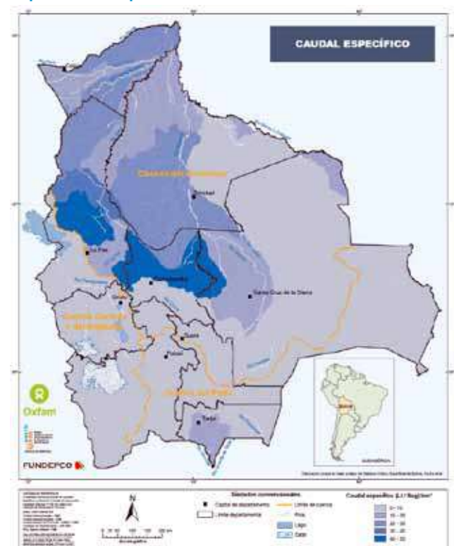
Mapa 5. Caudal Específico
