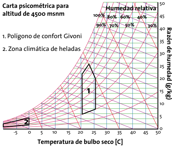
Figura 14. Carta psicométrica, altitud de 4 500 msnm
